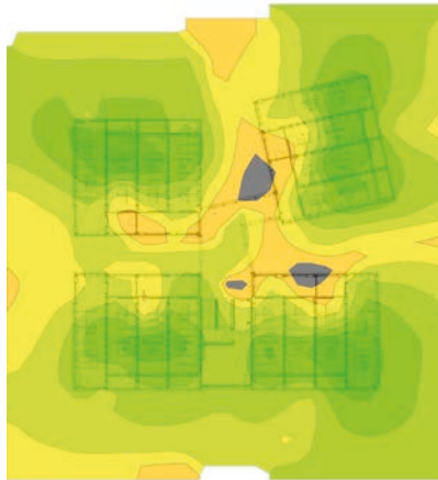
Abb. 2: Signalstärke 2,4GHz Frequenzband
